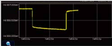
트렌드 표시
