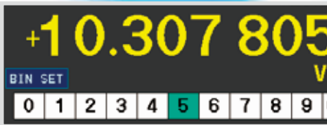
BIN 기능
