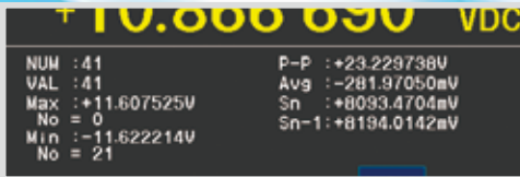
통계 표시
