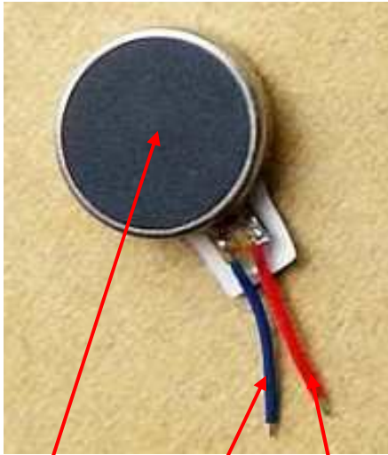
진동모터 전원 (-) (+)
