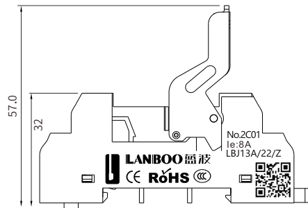
带测试扳手 Test wrench
