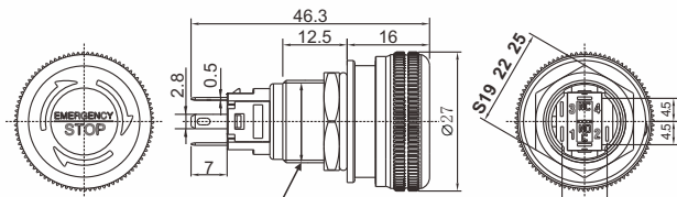
M16x1 M19x1 M22x1
