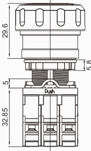
M1急停(塑料红色头部)
