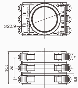
所有触点模块尺寸相同
