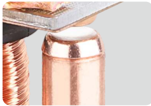
大银触点 Big Silver Contact
