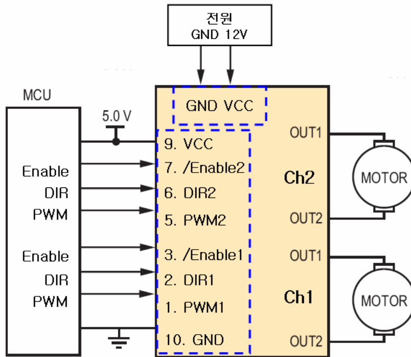
AM-DC2-2D 블록 다이어그램
