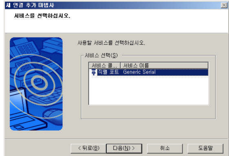
그림 3.5: “직렬포트” 선택
