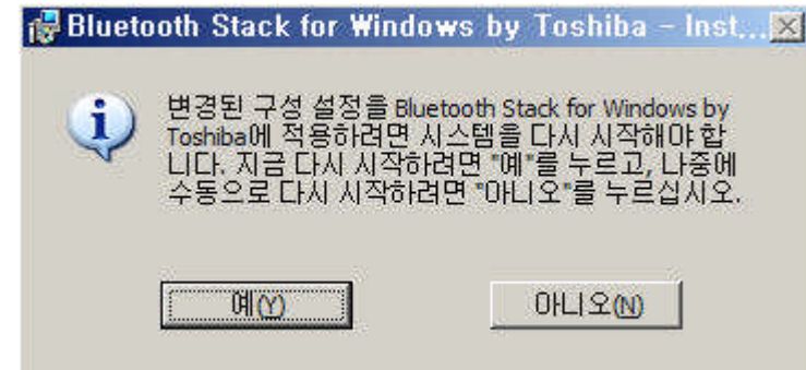
그림 2.6: 시스템 재시작
