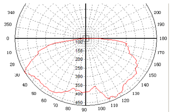
角度-光强 极坐标分布图
