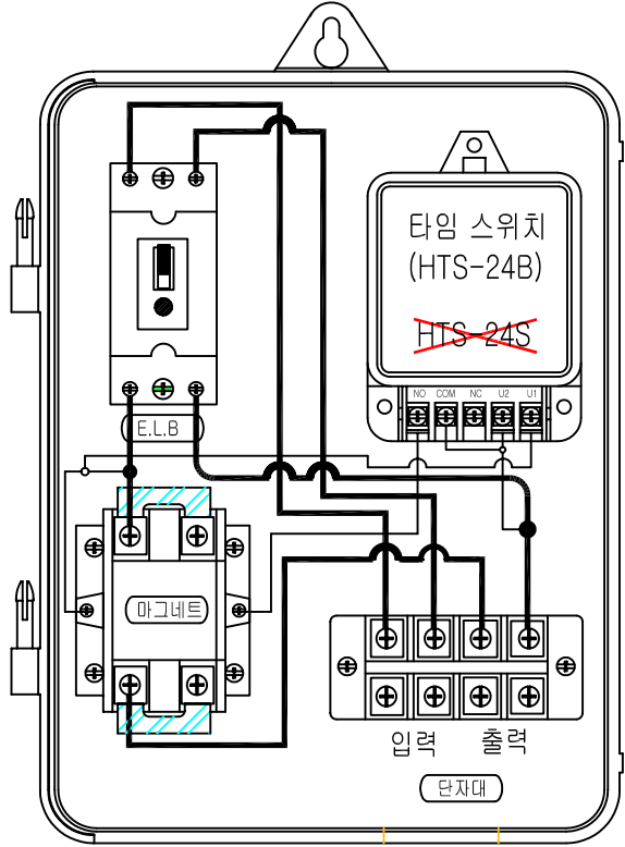
배치도 및 결선도
