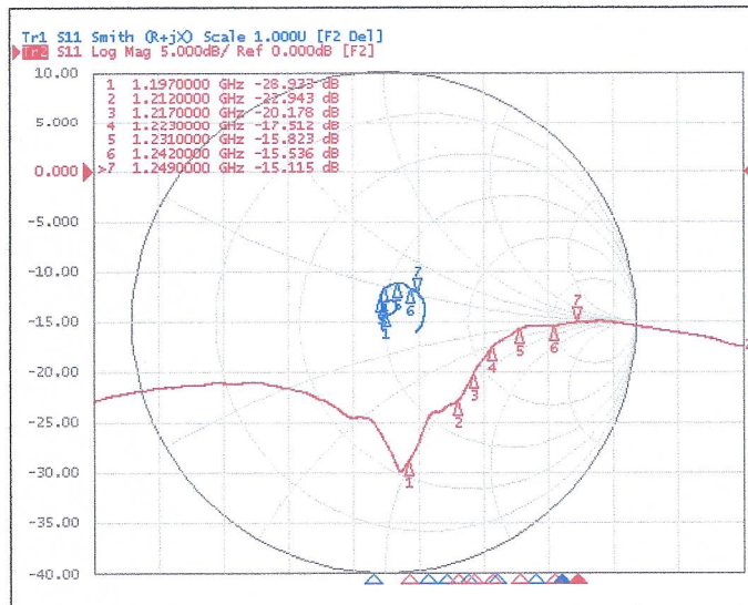
[Log mag & Smith Chart]
