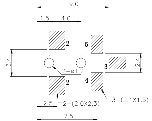
线路板开孔尺寸 P.C.B LAYOUT
