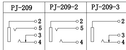
按点示意图 SCHEMATIC
