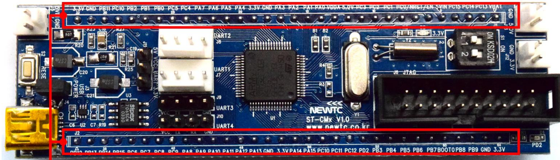
ST-CM3-A-MAIN 메인보드 및 브레드보드 실장용 커넥터
