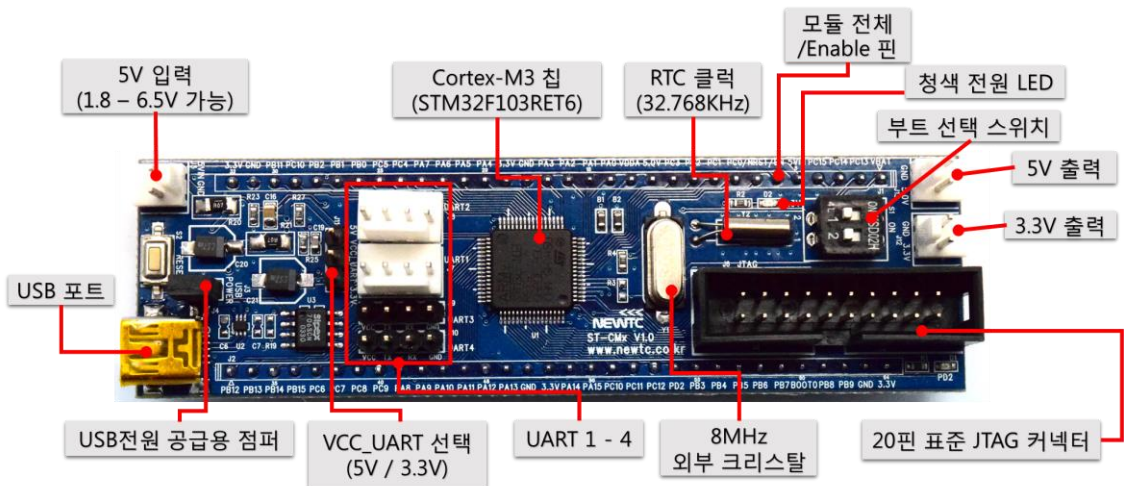
ST-CM3 V1.0 모듈 하드웨어 구성도
