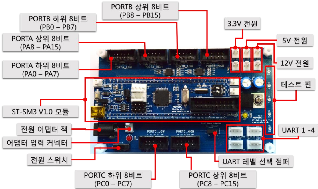
ST-CM3-A-MAIN V1.0 하드웨어 구성도
