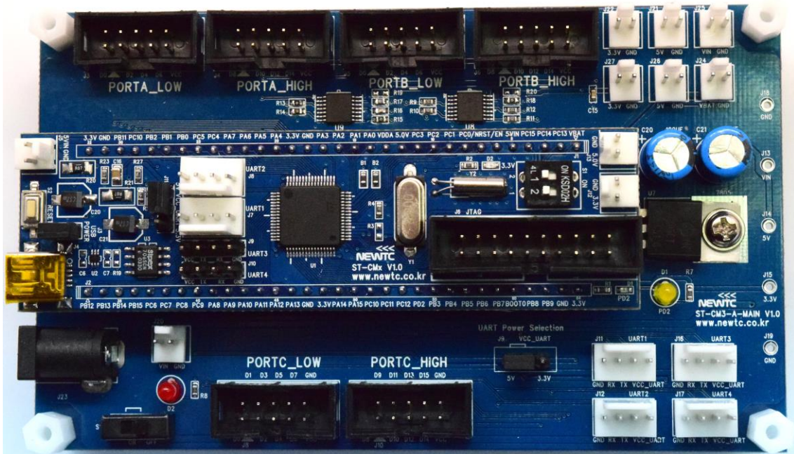
ST-CM3-A-MAIN V1.0 (ST-CM3 V1.0 이 장착된 모습)
