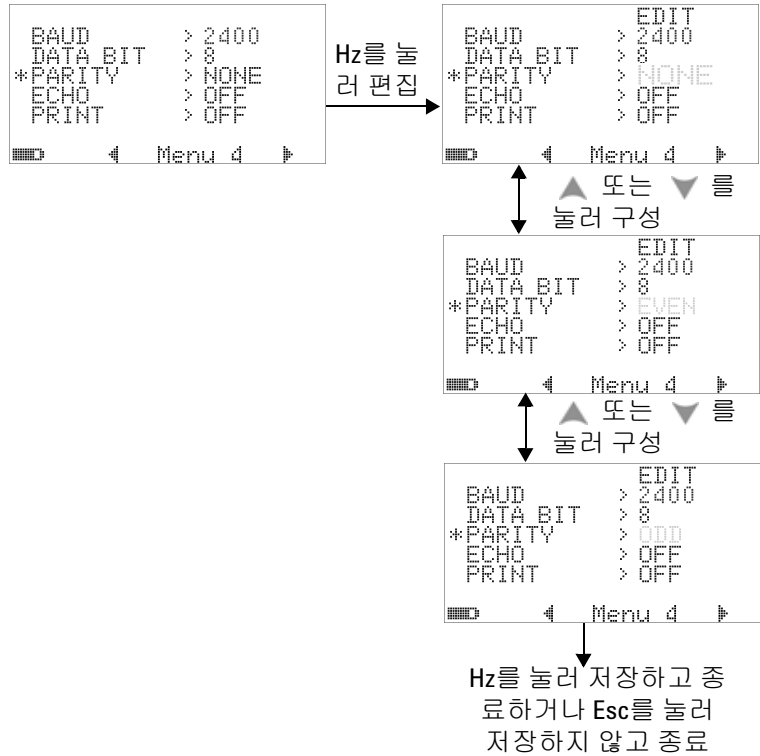
그림 4-19 원격 통신을 위한 패리티 검사 설정
