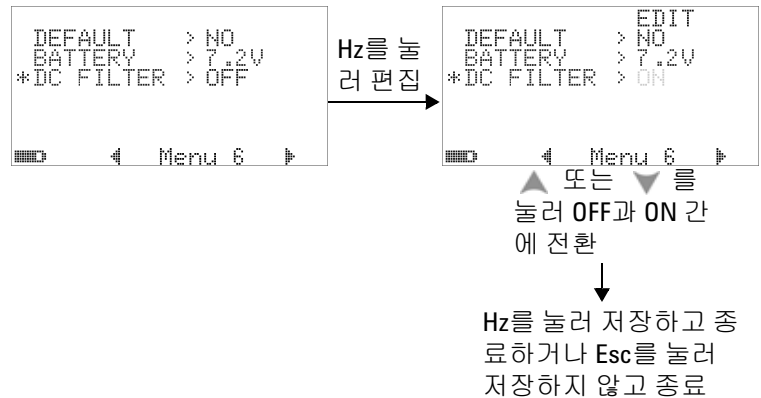
그림 4-32 DC 필터
