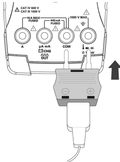
그림 2-16 멀티미터에 어댑터가 포함된 프로브 연결하기
