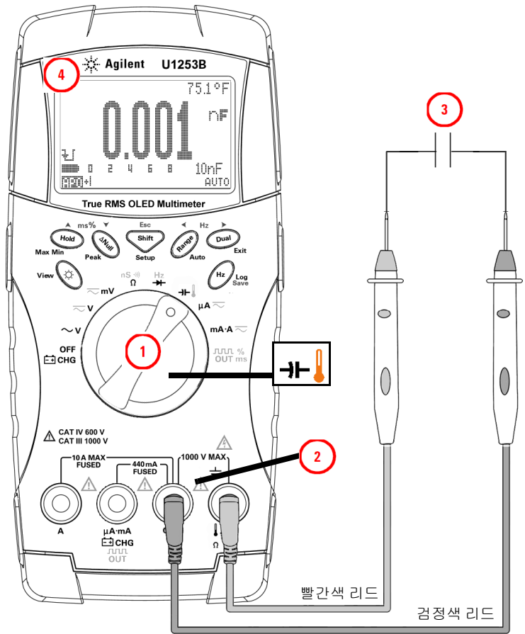
그림 2-14 캐패시턴스 측정
