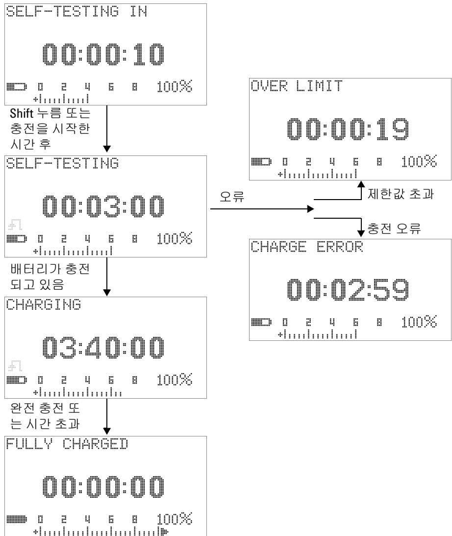
그림 5-7 배터리 충전 절차
