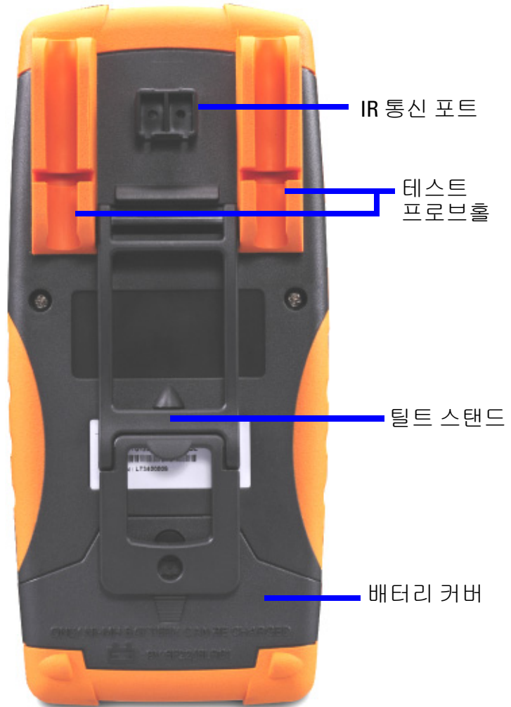
그림 1-5 후면판
