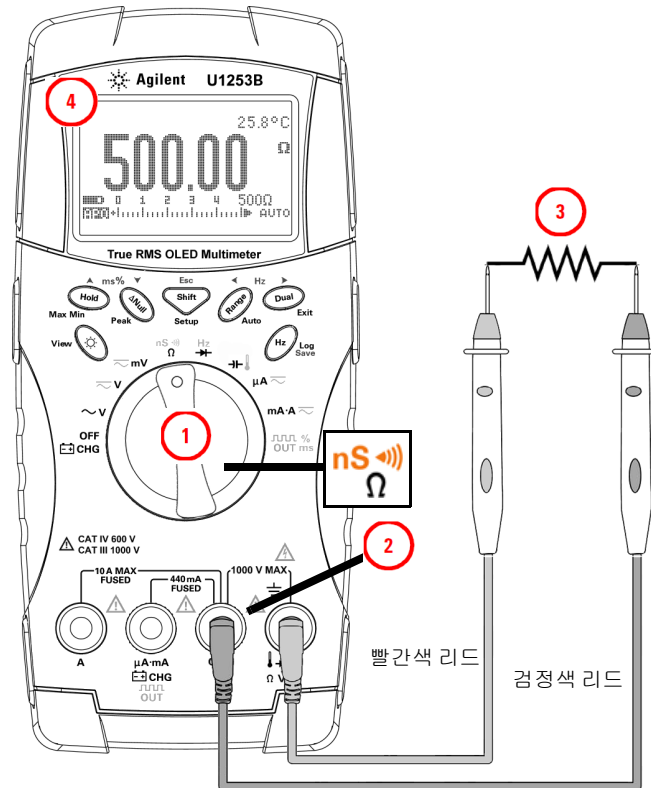
그림 2-8 저항 측정
