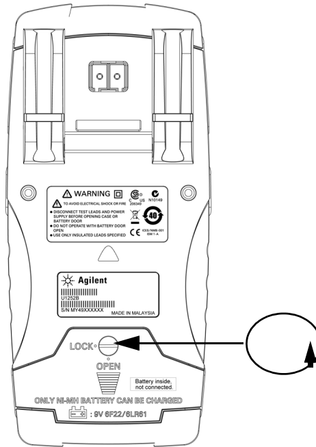
그림 5-2 Keysight U1253B True RMS OLED 멀티미터의 후면판
