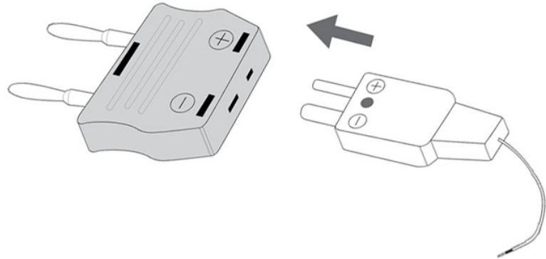
그림 2-15 비보상 전송 어댑터에 열 프로브 연결하기
