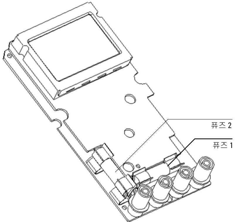
그림 5-9 퓨즈 교체
