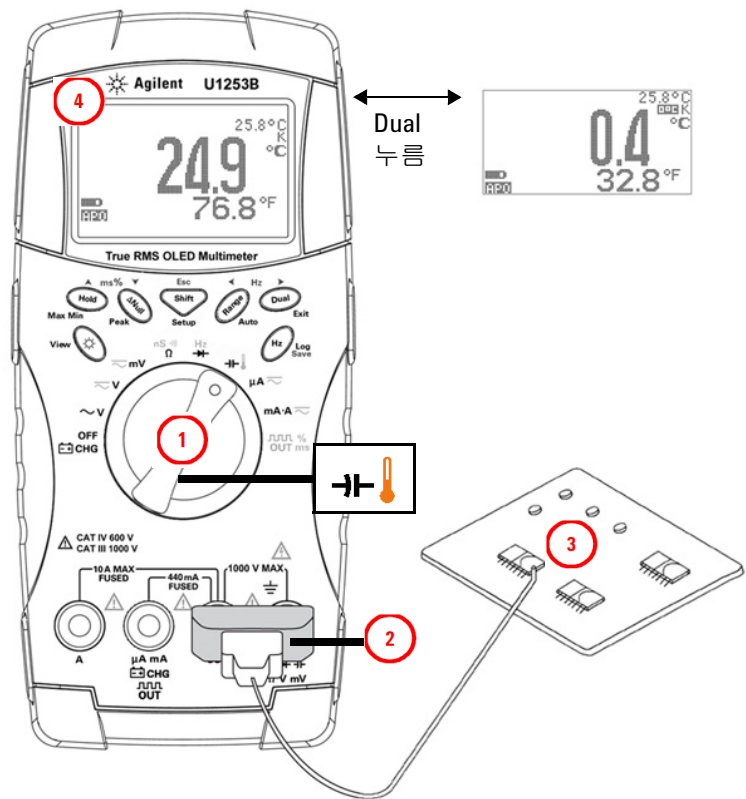
그림 2-17 표면 온도 측정
